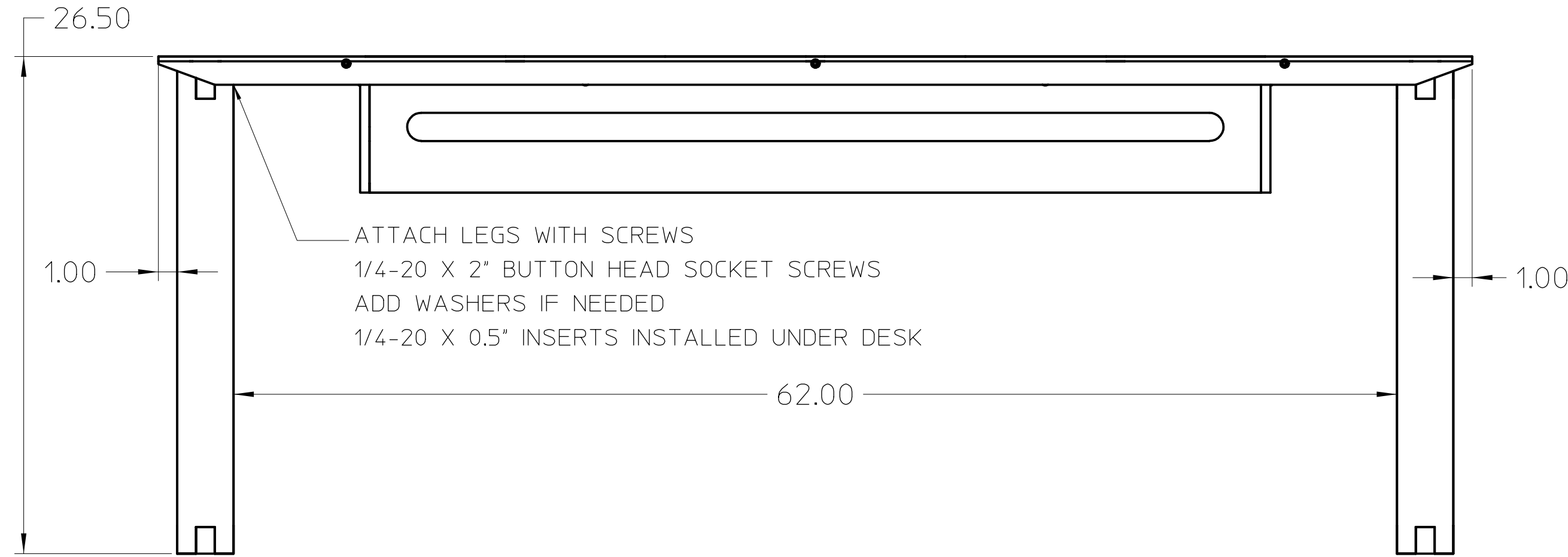
FRONT1 SCALE 1:6
